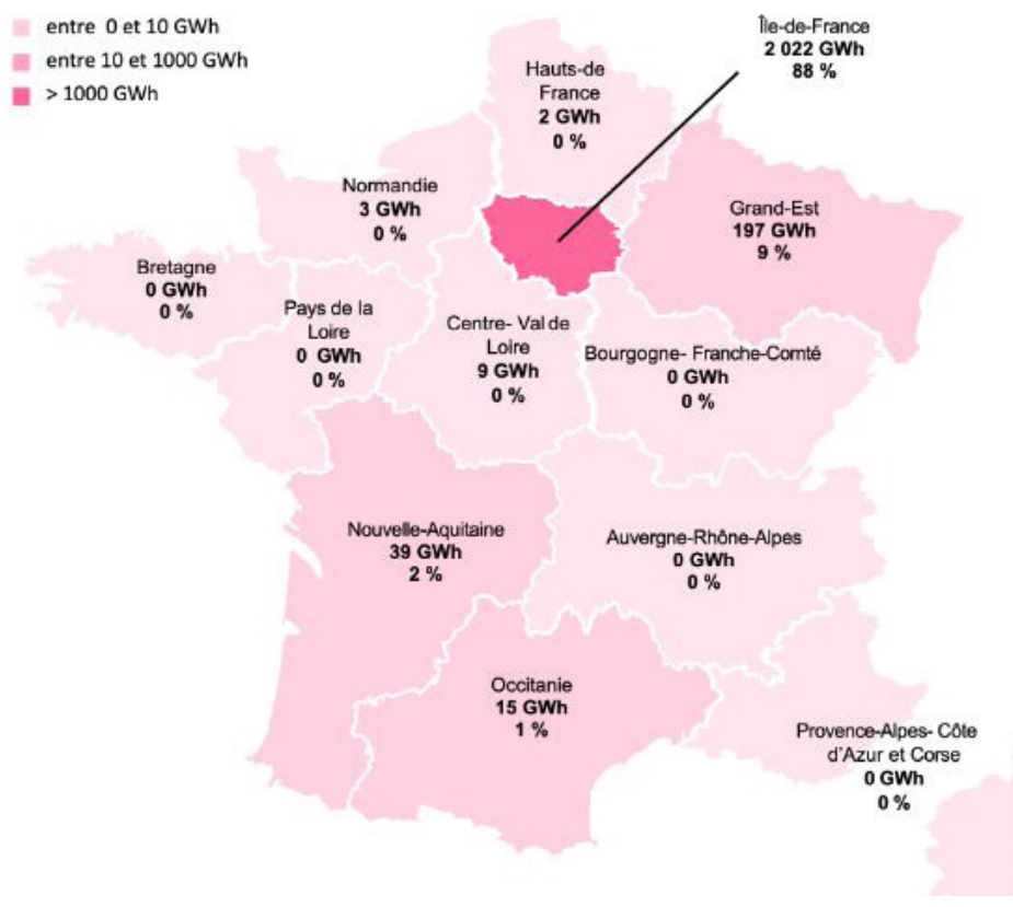
Figure 4 : production de chaleur issue de géothermie dans les réseaux de chaleur (géothermie directe, géothermie assistée par pompe à chaleur) en 2021. Source : Fedene/SNCU.
