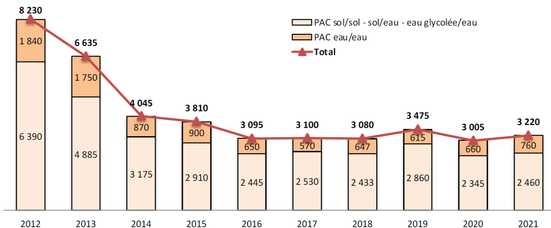
Figure 2 : évolution du nombre de pompes à chaleur géothermiques individuelles vendues en France de 2012 à 2021. Source : Observ'ER.
