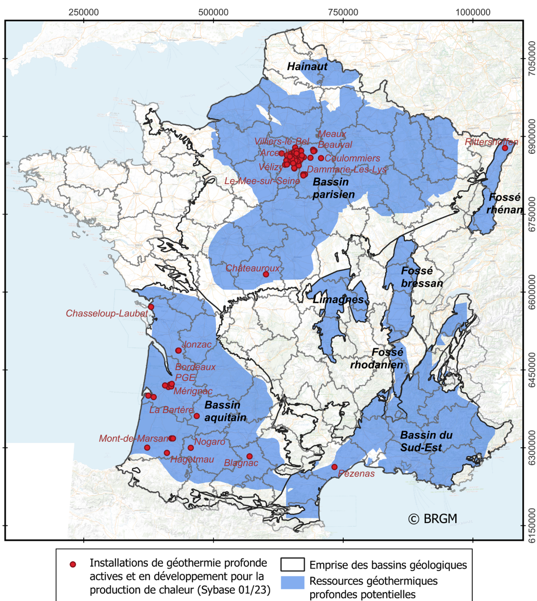
Figure 3 : aquifères profonds en France métropolitaine. Source : BRGM.
